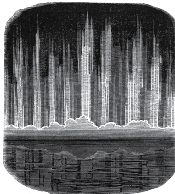
Aurore australe.
